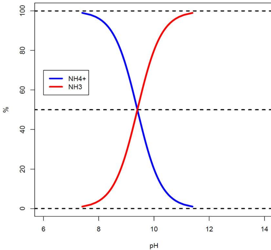
Figur 1: Figuren viser hvordan konsentrasjonen i prosent mellom uionisert, giftig ammoniakk ( \text{NH}_3 ) og ionisert, ugiftig ammoniakk ( \text{NH}_4^+ ) forholder seg til hverandre ved ulik pH. For å unngå ammoniakkforgiftning for fisk bør pH holdes ned mot 7,1 i pH. Figuren er hentet fra institutt for biovitenskap på Universitetet i Oslo.
