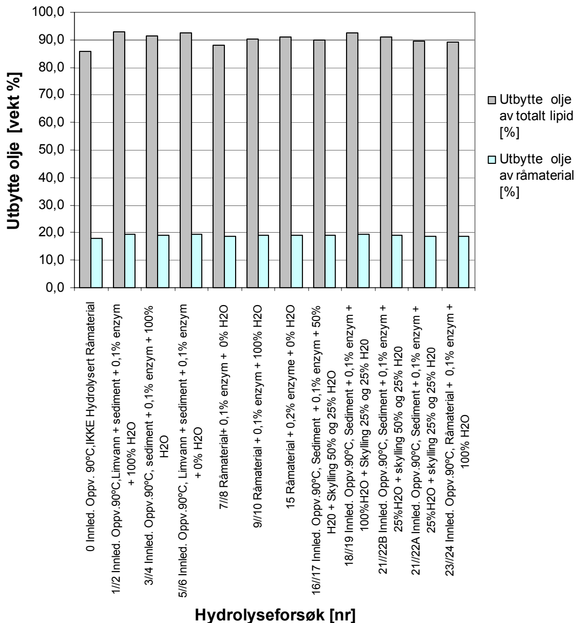
Figur 6. Resultat fra de ulike prosessalternativene, for utbytte av olje i både vekt % av totalt lipid tilgjengelig i råmaterial og i vekt % av våt vekt råstoff.
