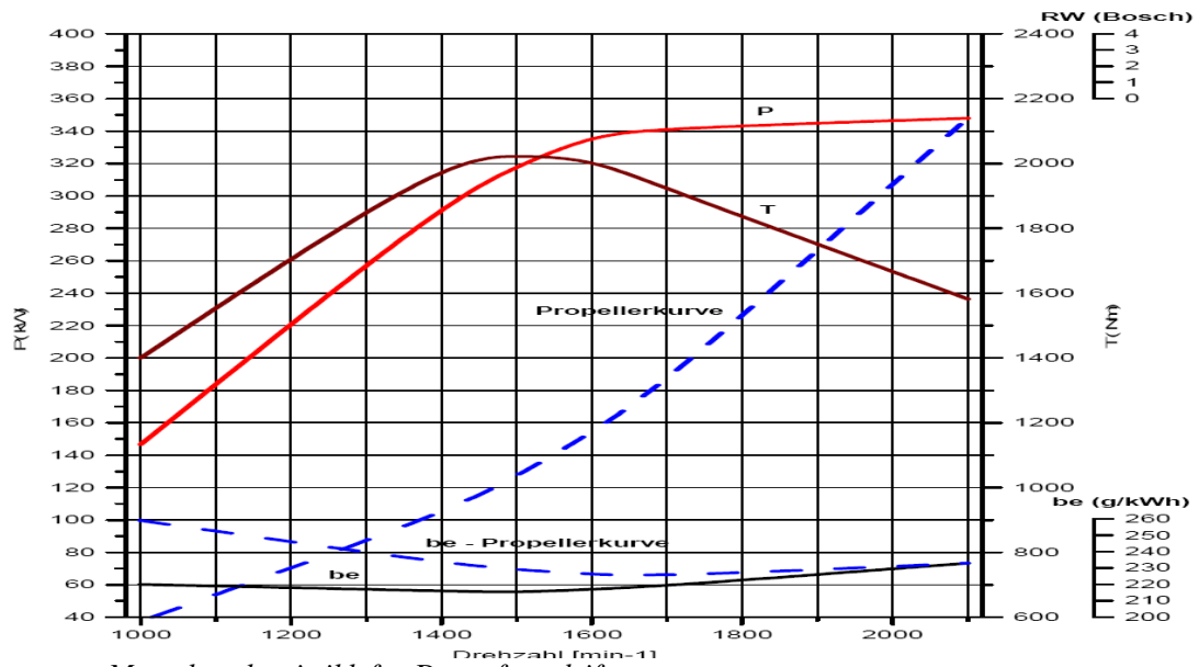
Motor karakteristik for Deutz framdriftsmotor
