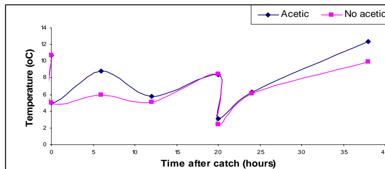
Figur 7. Temperatur i tanken hvor sild ble lagret
