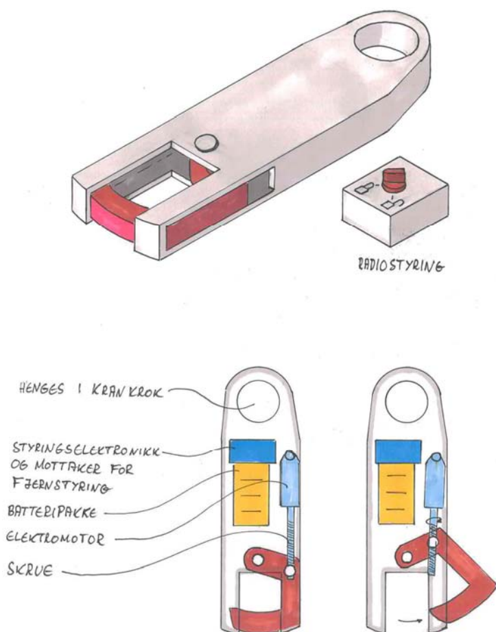
Figur 36. En mulig utforming av en fjernstyrt utlôsbar krok.
