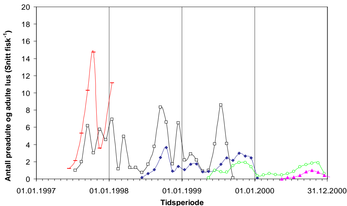
Figur 19. Månedsvise gjennomsnitt av antall preadulte og adulte lus per fisk i Nordland; Troms og Finnmark. Data er delt opp i ulike årganger av laks. 96 årsgang = røde fylte rektangler, 97 årsgang = åpne kvadrater, 98 årsgang = blå fylte romber, 99 årsgangen = grønne åpne sirkler, 00 årsgangen = rosa trekanter
