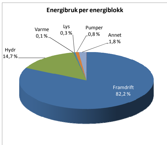
figur 16: Fordeling av energi på brukere fartøy 3
