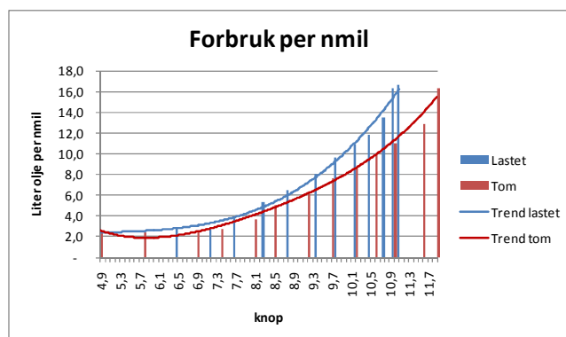
figur 67: Differanser i fremdriftseffektivitet med tom og lastet båt. Autolinefartøy med planende skrog.
