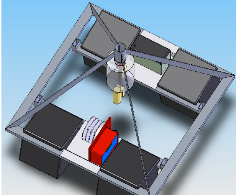
Figur 6 3D-illustrasjon av flåte (teget av Åstvedt Industri AS). Flåten holdes flytende av fire pontonger, en i hvert hjørne. Flåten bærer den styrbare vinsjen (BJ5000 fra Belatronic AS), et GSM-modem med styresystem og et bilbatteri. For å få balansert oppdrift står vinsjen på en side av flåten mens bilbatteriet står på motsatt side. Vinsjen drar målesonden opp og ned via en trinse festet i toppen av tårnet. Aluminiumsrammen er 1,5x1,5 m og 1m høy.
