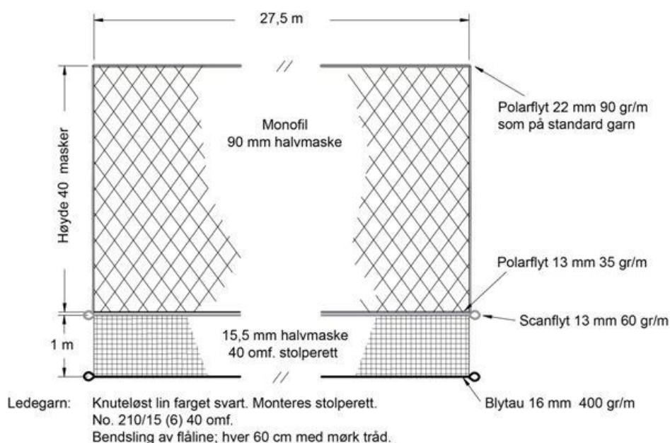
Figur 1. Torskegarn med notpanel.
