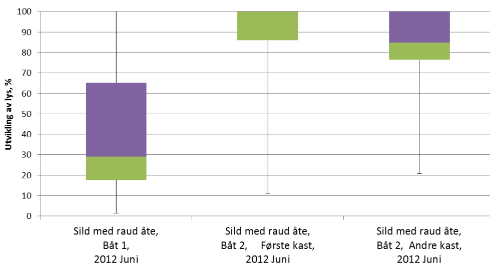
Figur 6. Enzymatisk aktivitet i nyfanget nordsjøsilde som ble målt en time etter fangst, inkubasjonstid i prøverøret var 1 time. Begge båter rapporterte samme mengde åte inn til auksjonen: 3. Box plot som viser kvartiler, median og utliggere i hver måling.
