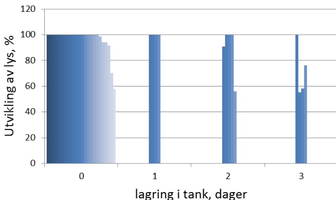
Figur 5. NVG silid. Prøvene ble tatt fra RSW tanken under lagring i opp til 3 døgn. Hver søyle representerer en enkelt prøvefisk.
