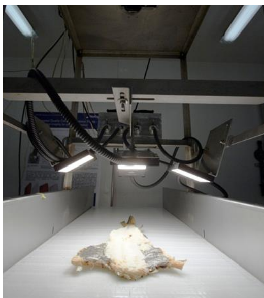
Bilde 2 Spektroskopisk måling av lyshet og gulfarge på klippfisk lagret ved 4 °C
