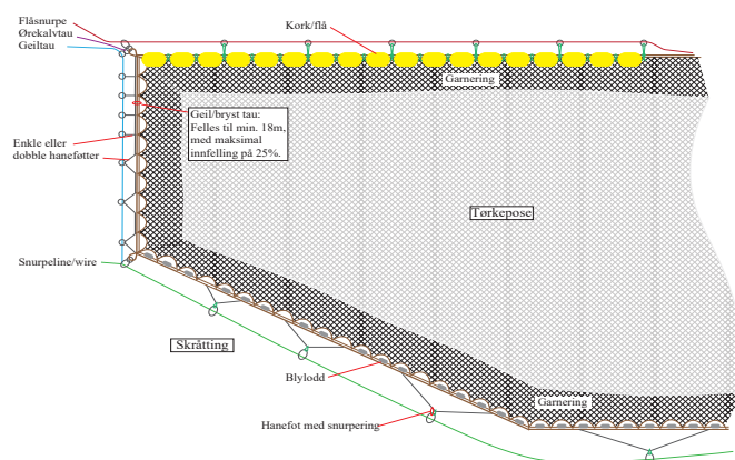
Figur 1: Rigging av geila slik det ble foreslått under Gardermoen-møtet. Notas lengde i brystenden skulle begrenses av et geil-tau på minimum 18 m og en maksimal innfelling langs geil-tauet på 25 %.
