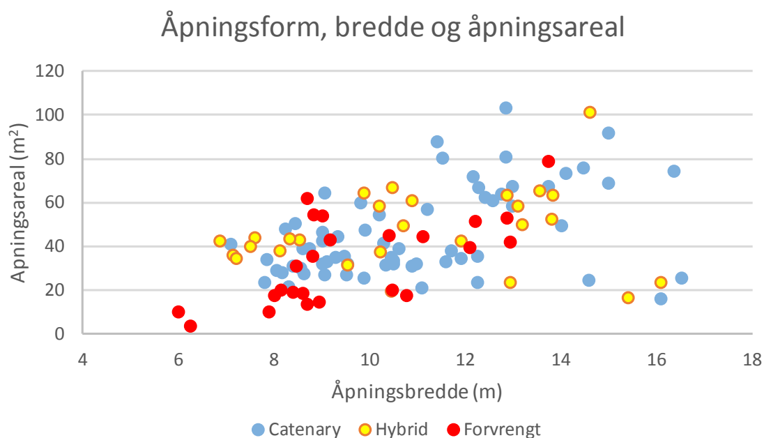
Figur 26. Utslippsåpningens vidde og areal ved tre ulike former: Kjedeflinje (=Catenary), hybrid og forvrent form.
