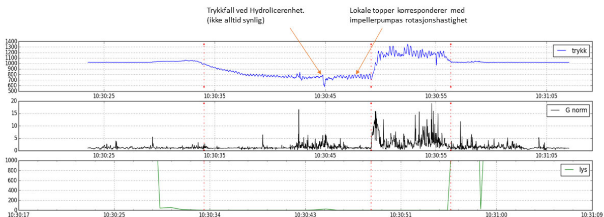
Figur 28 - Eksempel på data fra sensorfisk. Her synes hydrolicerenhetene tydelig som en endringer i trykkkurven (øverst). Trykkvariasjonene fra impellerpumpa synes også som overliggende signatur. Nederst er lyskurven, som kun ble benyttet til lokalisering av sensorfiskene. Ved starttidspunkt (1. røde strek) er lyset registrert lik null, med en liten forhøyning midt i forløpet når sensorfisken passerer fisketelleren. Ved slutten av forløpet registreres det umiddelbart mye lys når sensorfisken kommer ut på silkassen. Fra avlusing 2.
