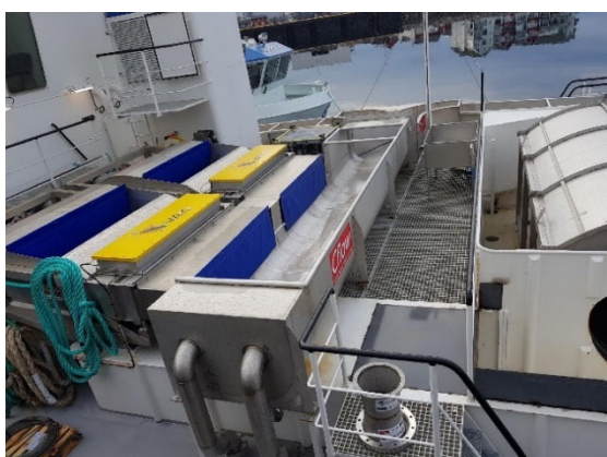
Figur 20 – Utløpssiden på Hydrolicer LH2245 Hydroflow. Fisken telles etter pumping (doble ejetorpumper) med Vaki fisketellere (gule lokk) før avluset laks kommer ut i rennen fylt med vann for overføring til merd. Posisjon 2: Fisk for lustelling, evaluering av stress og velferdsscore ble håvet ut på utløpssiden og overført til kar plassert ved rennen (høyre bilde).
