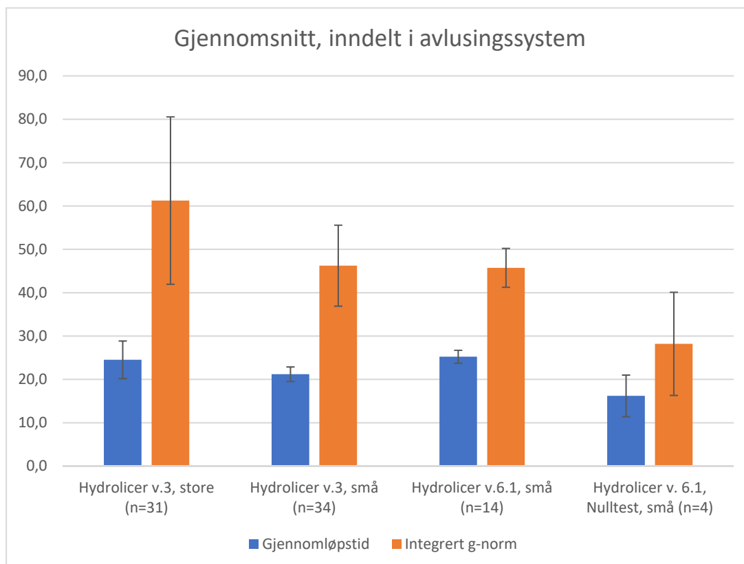
Figur 26 - Gjennomsnitt av gjennomløpstid og integrert g-norm inndelt i avlusingsssystem. Data fra stor type sensorfisk i Hydrolicer versjon 6.1 er utelatt på grunn av lav N (2). "Nulltest" er gjennomløpstid for sensorfiskene når enhetene for avlusning ikke var innkoblede.
