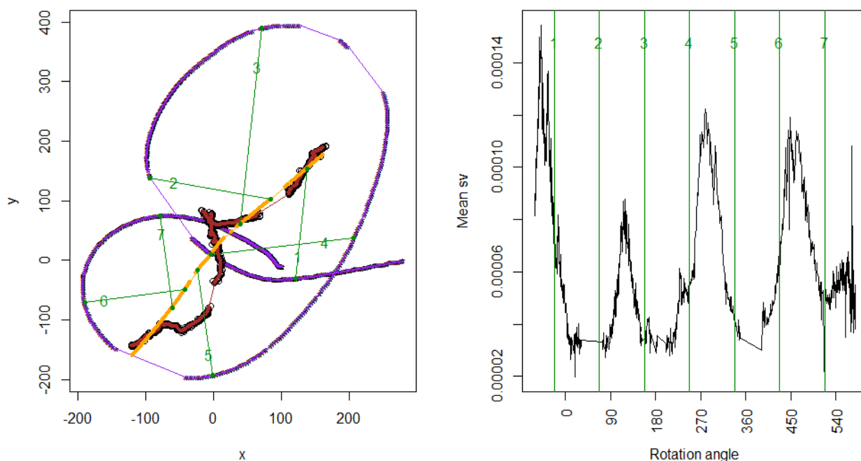
Figur 10. Til venstre: Båtens posisjon i lilla, stimens senterpunkt i rødt og glattet stim svømmeretning i gult. De grønne linjene og tallene viser innfallsvinkel. Til høyre: Ekkostyrke (sv m-1) i forhold til rotation angle (1. runde = 1 - 360°, 2. runde = 361 - 720°). De grønne strekene og tallene viser relativ posisjon for båt og stim.
