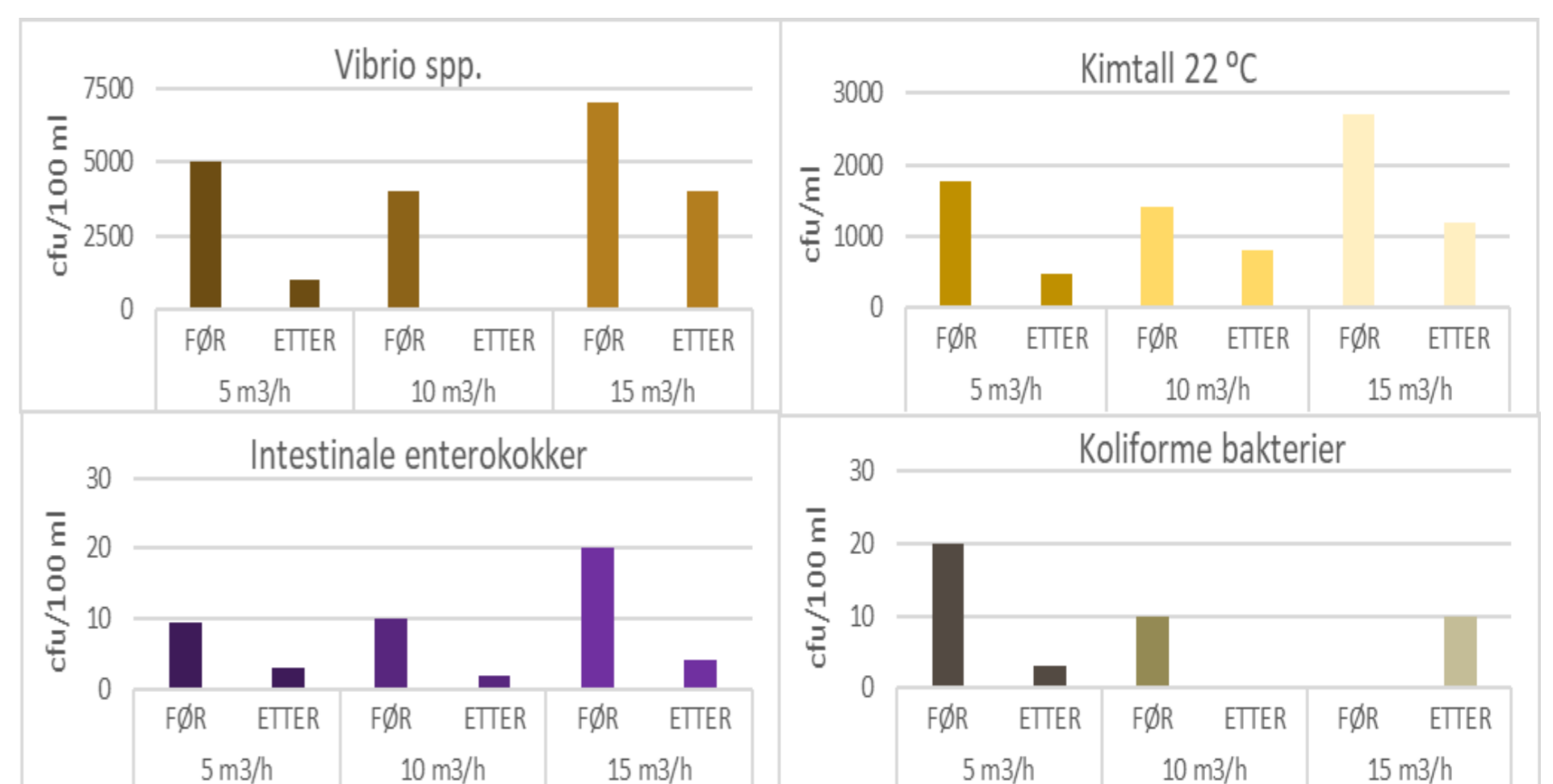
Figur 2: Bakteriologisk vannkvalitet i RSW-kjølt blodvann før og etter sentrifuge ved ulike fødehastighet.
