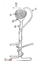
Fig. 3. Ekskresjonssystemet = nefron. a glomerulus, b blodåre til c blodåre fra, d Bowmans kapsel, e proximale tubulus, f distale tubulus, g samlerør (ref. Amin m.fl. Histologisk Atlas)
