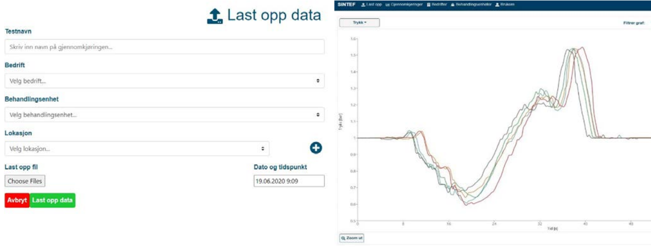
Figur 5: Skjermbildeeksempler fra brukergrensesnitt. Figuren til høyre viser sammenligning av flere trykkkurver, mens bildet til venstre viser menyer for opplasting av data.
